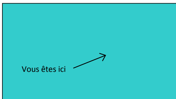
Résumé de l'épisode précédent par une illustration inutile : Orival entre -96 et -72 millions d'années Echelle 1/50000ème
